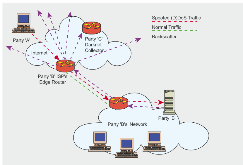
Rysunek 5. Przykład rozproszenia wstecznego w przypadku ataku DDoS
