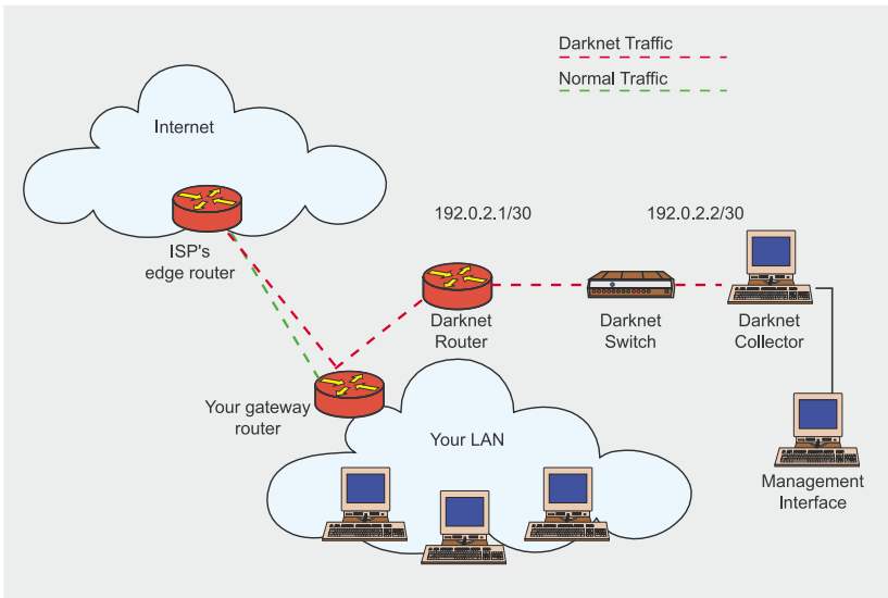
Rysunek 4. Referencyjna logiczna topologia sieci typu darknet
